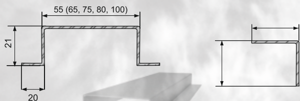
Профиль "П"-образный 55 (65, 75, 80, 100)х21.5х20х1.0 (1.1; 1.2)
