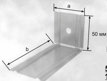
Кронштейн
